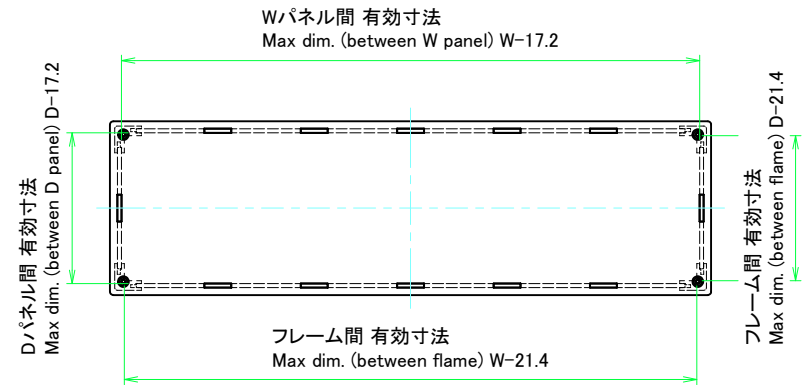
下カバー / Bottom cover
